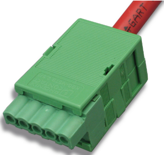
Abbildung 32: Montiertes CC-Link Kabelgehäuse
