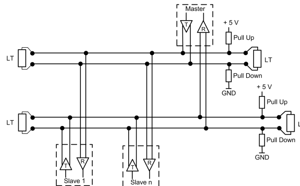
Abbildung 34: RS-422-Kabel
