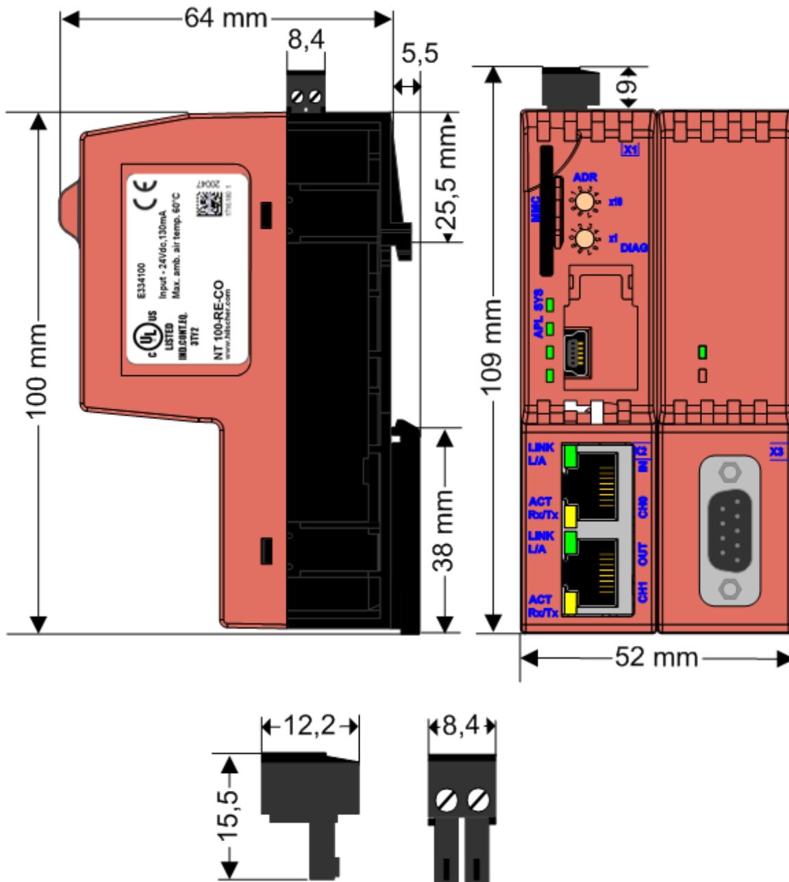
Abbildung 4: Abmessungen
