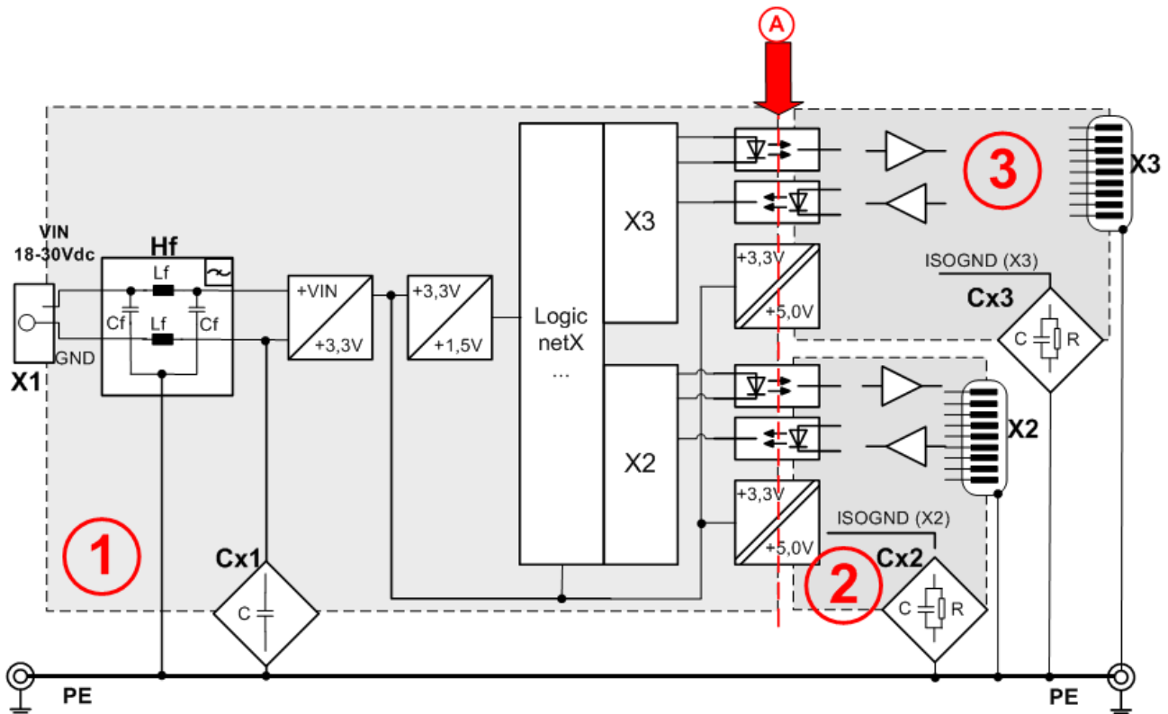
Abbildung 9: Galvanische Trennung NT 100-DP-XX / NT 100-CO-XX / NT 100-DN-XX-Geräten
