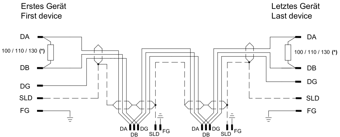
Abbildung 30: CC-Link-Kabel
