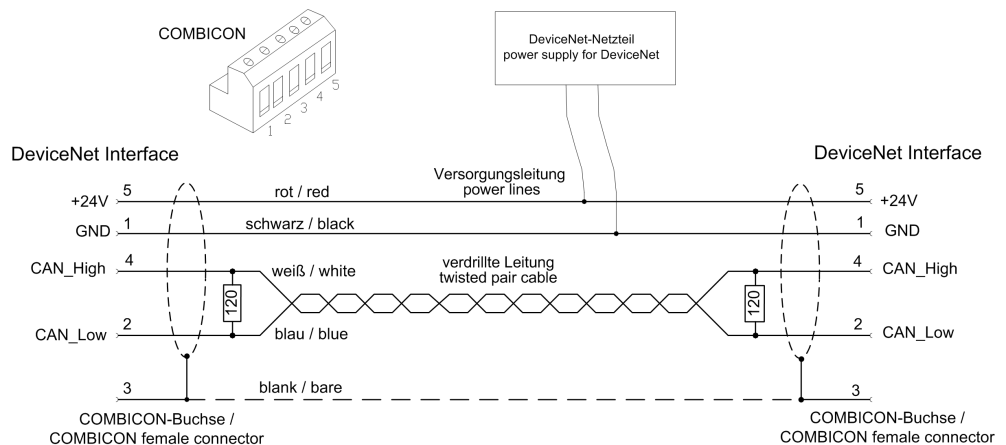
Abbildung 29: DeviceNet-Kabel und Terminierung
