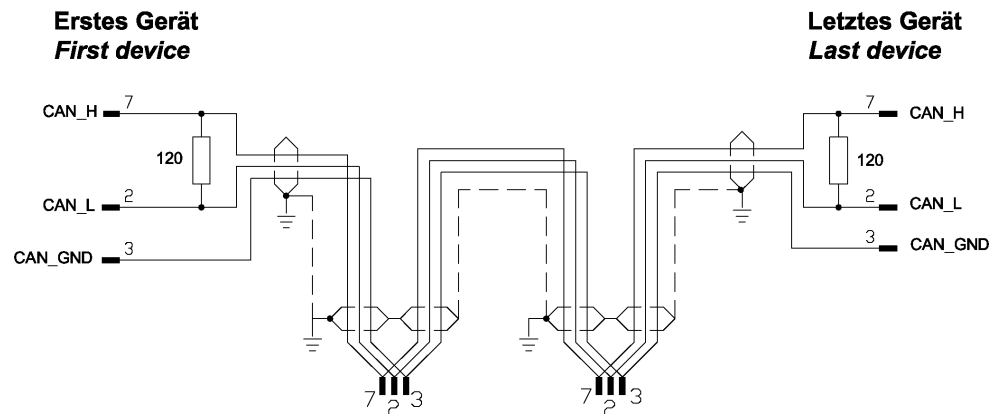
Abbildung 28: CANopen-Kabel und Terminierung
