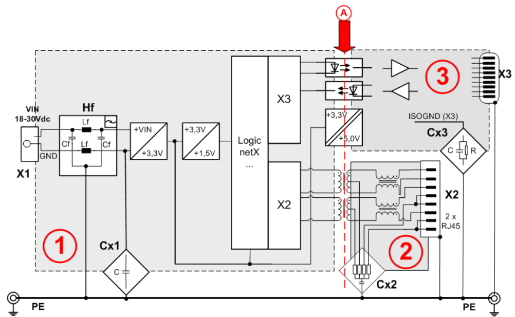
Abbildung 8: Galvanische Trennung NT 100-RE-XX-Geräte
