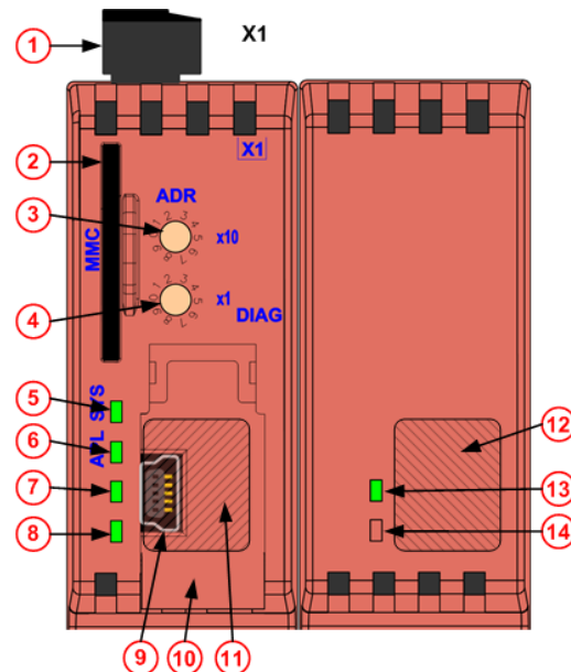
Abbildung 5: LEDs und Bedienelemente (obere Gerätehälfte)
