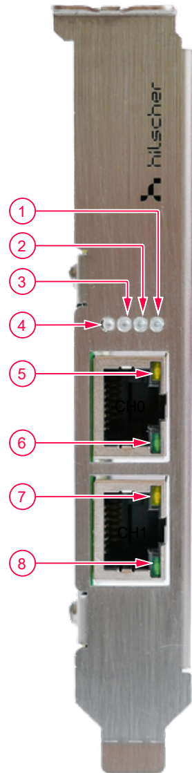
Abbildung 2: Slotblende und LED-Positionen
